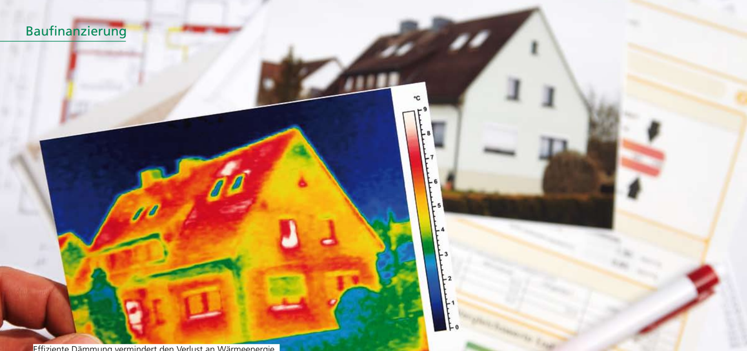
Effiziente Dämmung vermindert den Verlust an Wärmeenergie.
